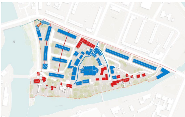
Abbildung: Baustufen des Wärmenetzes und Kennzeichnung der anzuschließ. Gebäude
